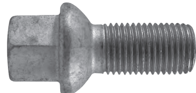
561-516 M14 x 1.5R x 36mm 17mm Hex
