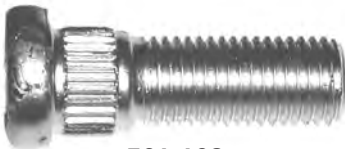
561-108 M12 x 1.5 x 38mm Knurl diameter: 14.3mm (Code M.1.0)
